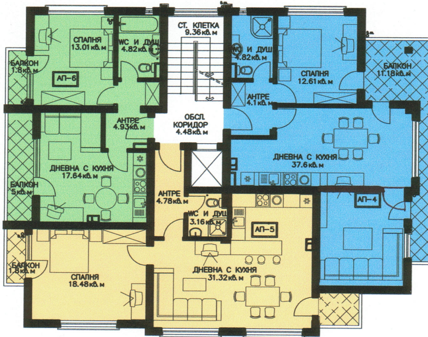
РАЗПРЕДЕЛЕНИЕ ПЪРВИ ЖИЛИЩЕН ЕТАЖ ЗП 215,3кв.м
