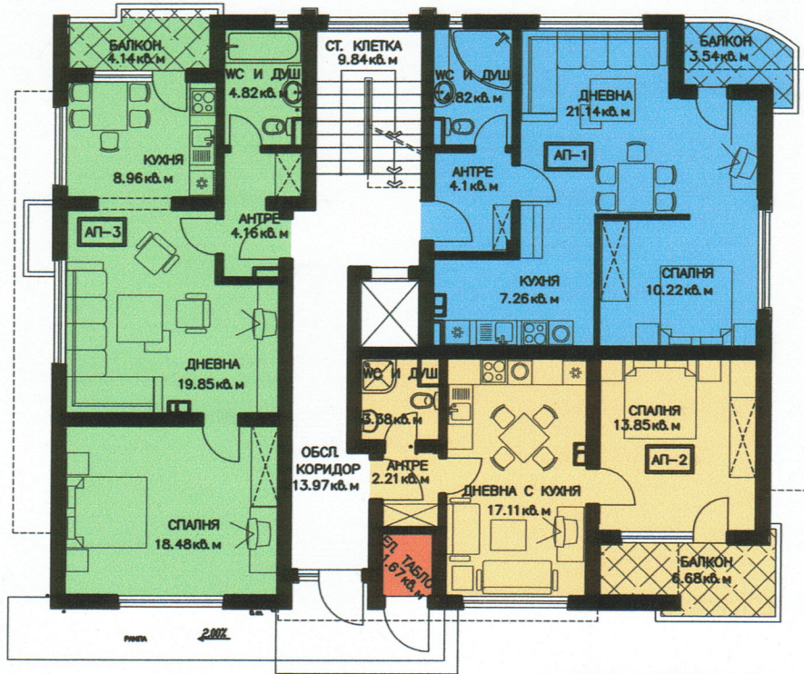
РАЗПРЕДЕЛЕНИЕ ПЪРВИ ЖИЛИЩЕН ЕТАЖ ЗП 215,3кв.м
